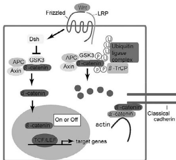
図 Wnt/ \beta -catenin経路と細胞間接着における \beta -cateninの役割。Wntシグナル非存在下では細胞質中の \beta -cateninはGSK 3によりリン酸化され、ユビキチンが結合してプロテアソームにより分解されるが、Frizzled受容体にWntが結合するとGSK 3 (glycogen synthase kinase 3 \alpha ) の働きは阻害されるので \beta -cateninは分解を免れ、核へ移行してTCF/LEFファミリーの転写因子と結合して、標的遺伝子の発現を活性化 (場合によっては不活性化) する。 \beta -cateninはWnt/ \beta -catenin経路の因子として働くだけでなく、細胞接着分子cadherinと結合して細胞間接着にも関与する。
