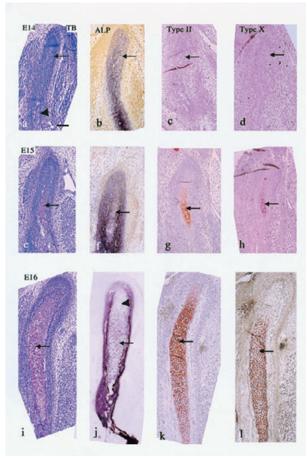
図2 胎齢14 (E14: a-d) と15 (E15: e-h) および16日齢 (E16: i-l) のマウス下顎頭軟骨の冠状断切片 (関節突起の長軸に平行な断面)。トリルイジンブルー染色 (a, e, i) とアルカリフォスファターゼ染色 (b, f, j)。さらに抗タイプIIコラーゲン抗体 (c, g, k) と抗タイプXコラーゲン (d, h, l) 抗体による免疫染色。
