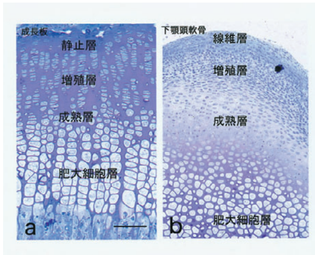
図1 3週齢ラット脛骨成長板(a)と下顎頭軟骨(b)
